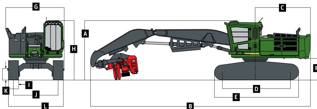
Ébrancheuse-tronçonneuse 3156G – cabine à entrée latérale
